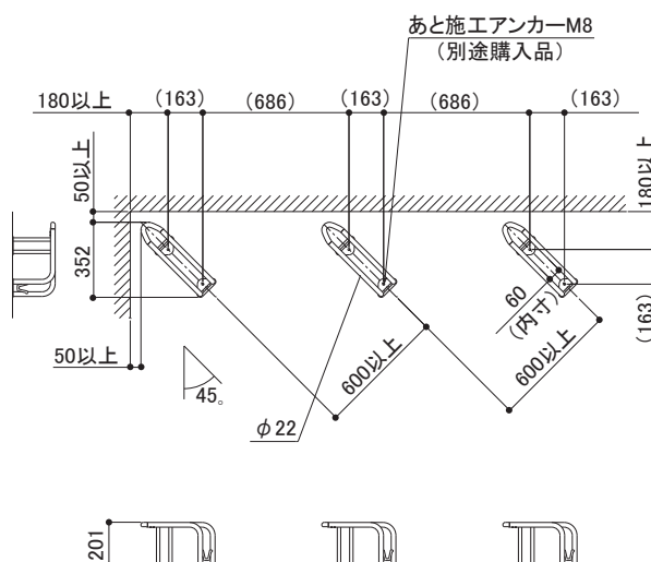
平置式3台(45°設置)の場合
