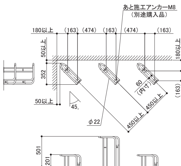
段差式3台(45°設置)の場合
