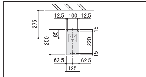
支柱ベースプレート部(90°設置の場合)
