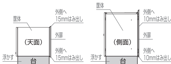
宅配ボックスを寝かせて配置し真横から見た図
