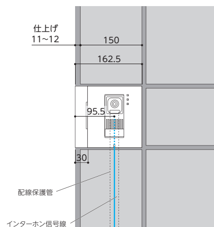
【参考施工図】 WAL-12
