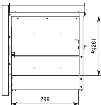
▼ 正面図(全開) 取出口寸法
