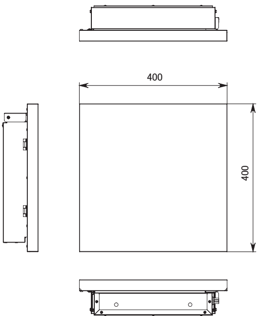
▼ 正面図(全開) 取出口寸法
