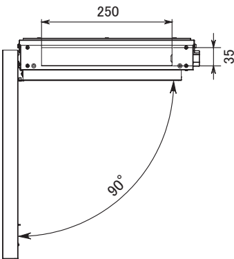
▼ 上面図(全開) 投入口寸法
