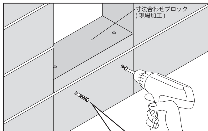
②コンクリートに下穴を開け、オールプラグボルトを取り付けます。(4ヶ所) 下穴：φ11mm 深さ40mm
