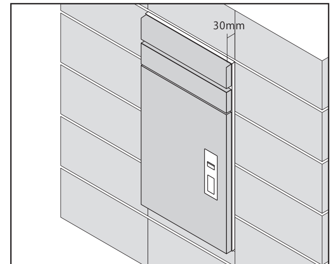
②扉開閉のかぶりを確保するため、壁の化粧面から30mm前へ出してください。
