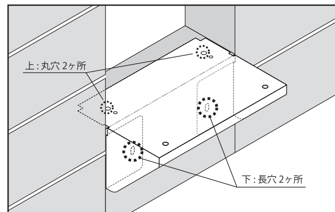
①台座を仮置きし、穴位置をマーキングします。(4ヶ所)
