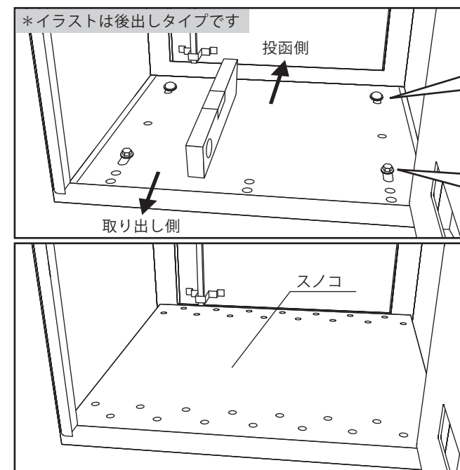
③水準器で確認しながら、底面のビス(ワッシャーを入れて下さい)を増し締めした後、スノコを戻します。
