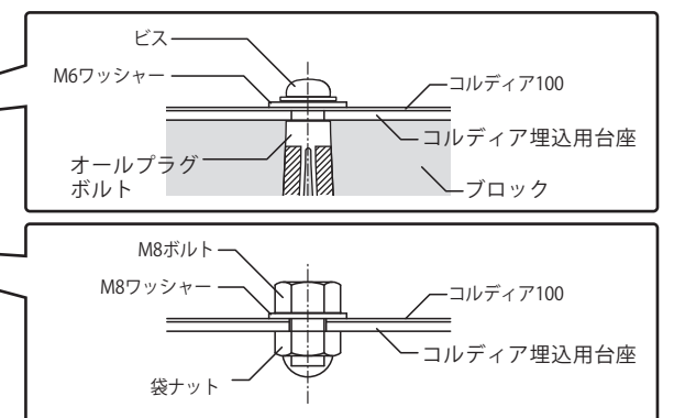
②扉開閉のかぶりを確保するため、壁の化粧面から30mm前へ出してください。
