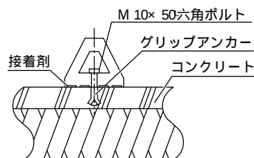
①部詳細(側面図)
