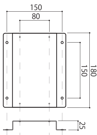
取付金具アンカーポイント図
